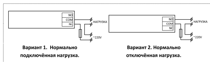
Рис.3 Схема подключения.
