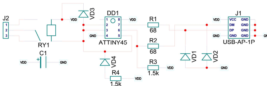
Рис. 2. Схема электрическая принципиальная
