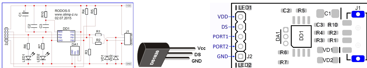
Рис. 2. Схемы электрическая принципиальная и монтажная
