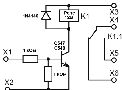
Рис. 4. VM146 (упрощённая схема).
