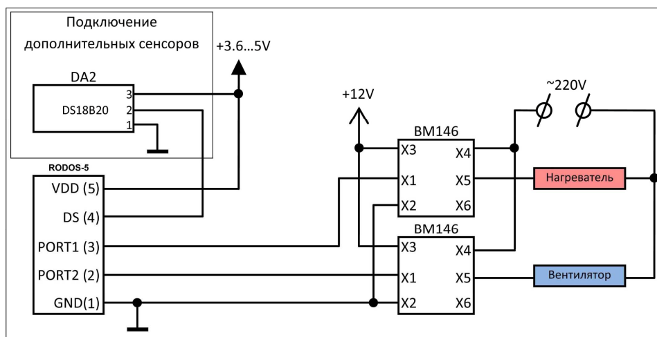
Рис. 3. Подключение дополнительных устройств.
